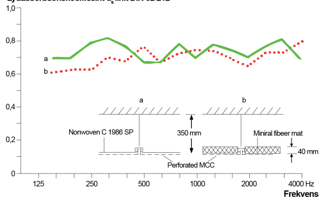
Lydabsorptionskoefficient \alpha_s i.h.t DIN 52 212
