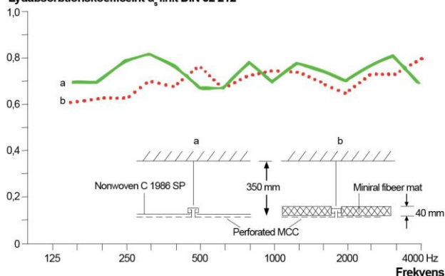
Lydabsorptionskoefficient \alpha_s i.h.t DIN 52 212
